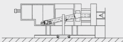
Posizione del nastro parallela alla pressa. Parallel position of the conveyor respect the moulding machine.
